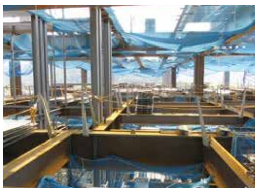
鉄骨工事 建方状況
