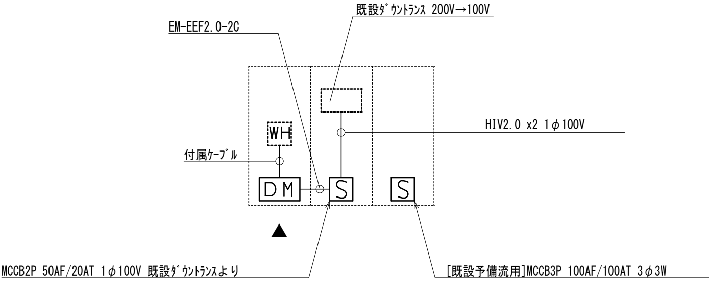
キュービクル詳細図
