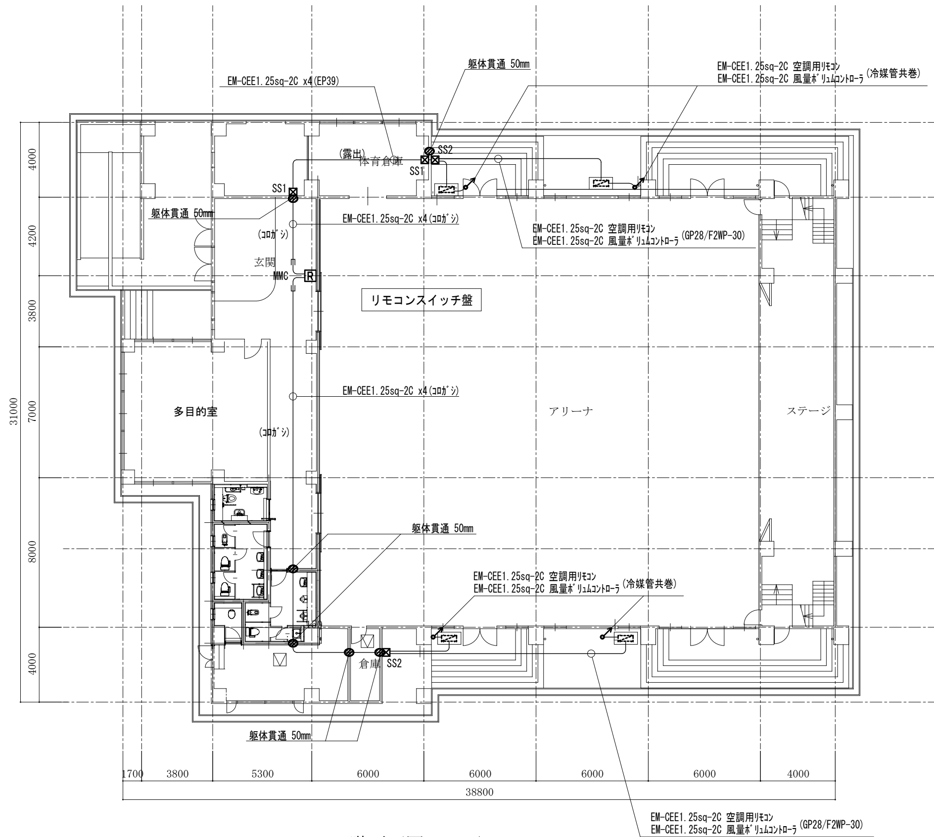
1階平面図 S=1/200
