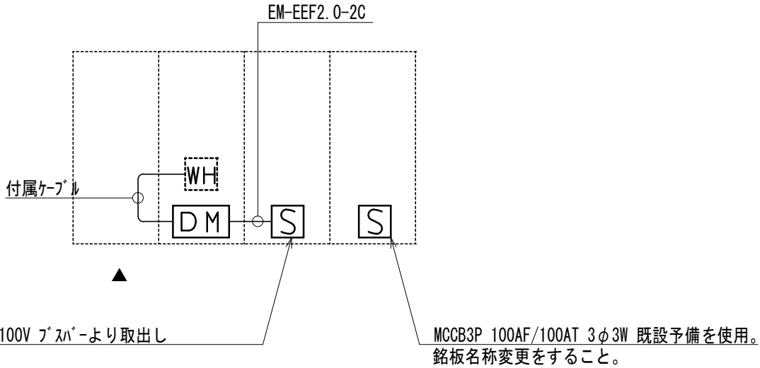
キュービクル詳細図
