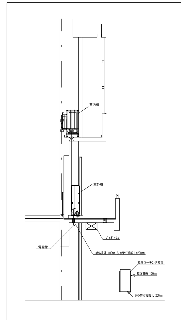
★ 貫通処理詳細図
