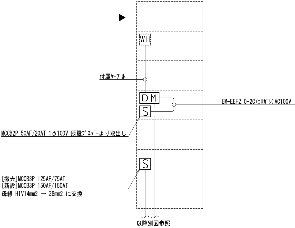
電気室詳細図
