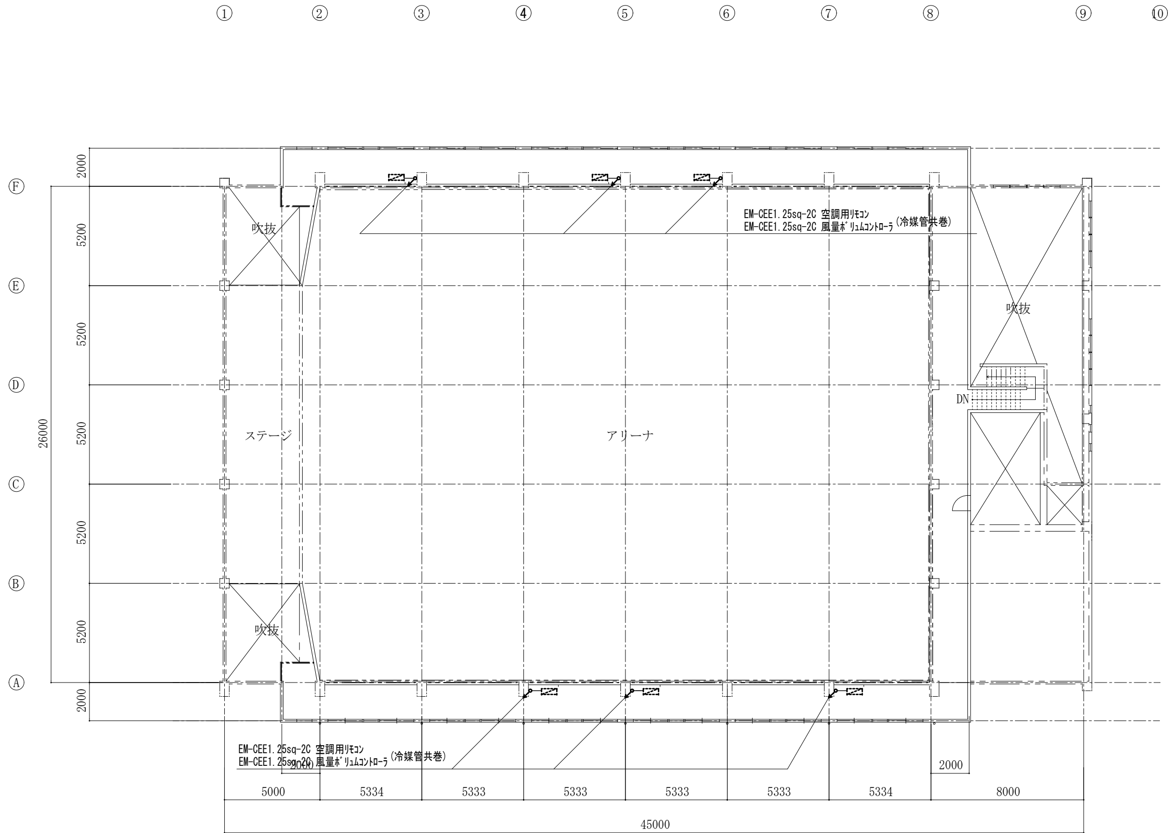
メンテナンスデッキ平面図 S=1/200
