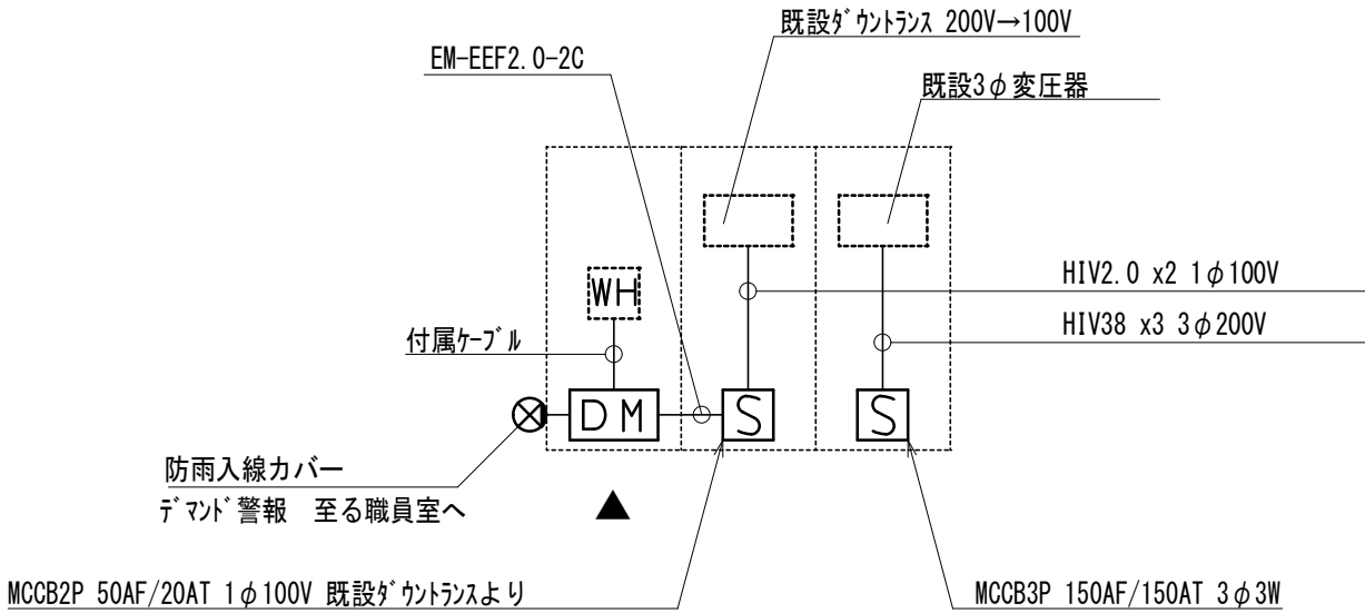
キュービクル詳細図
