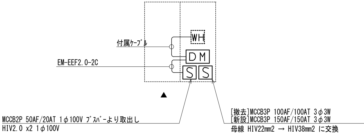
キュービクル詳細図
