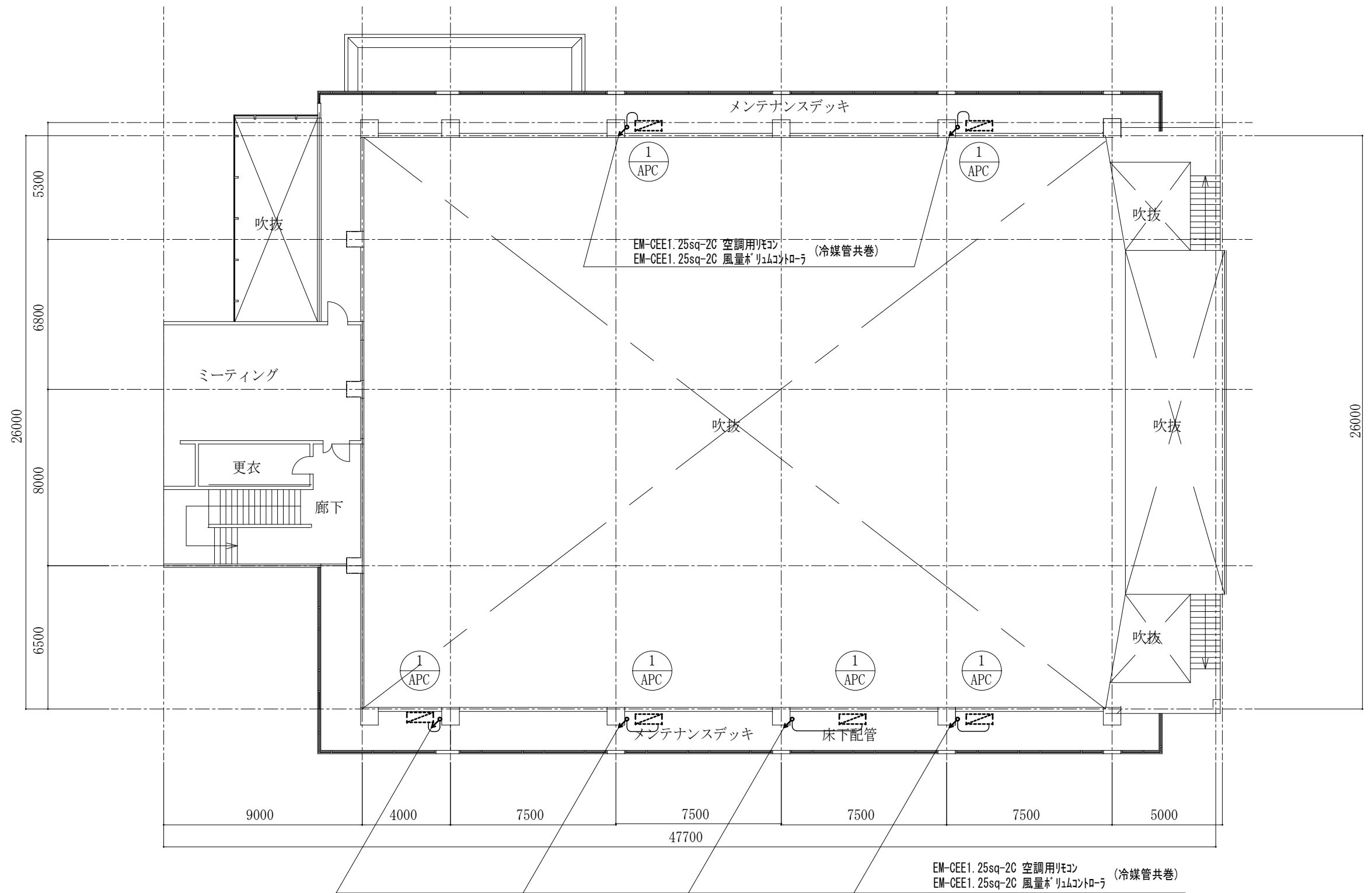
メンテナンスデッキ平面図 S=1/200
