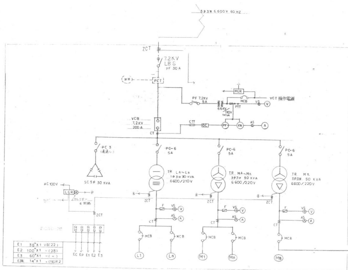
受変電設備 単線結線図
