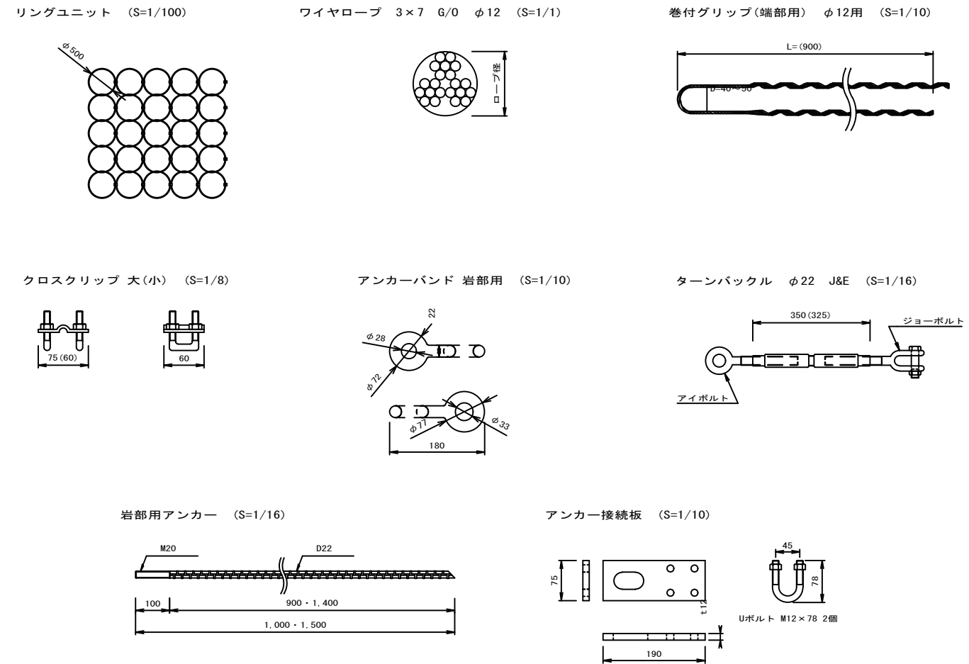
【使用部品図】
