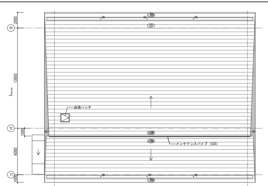
屋根伏図
